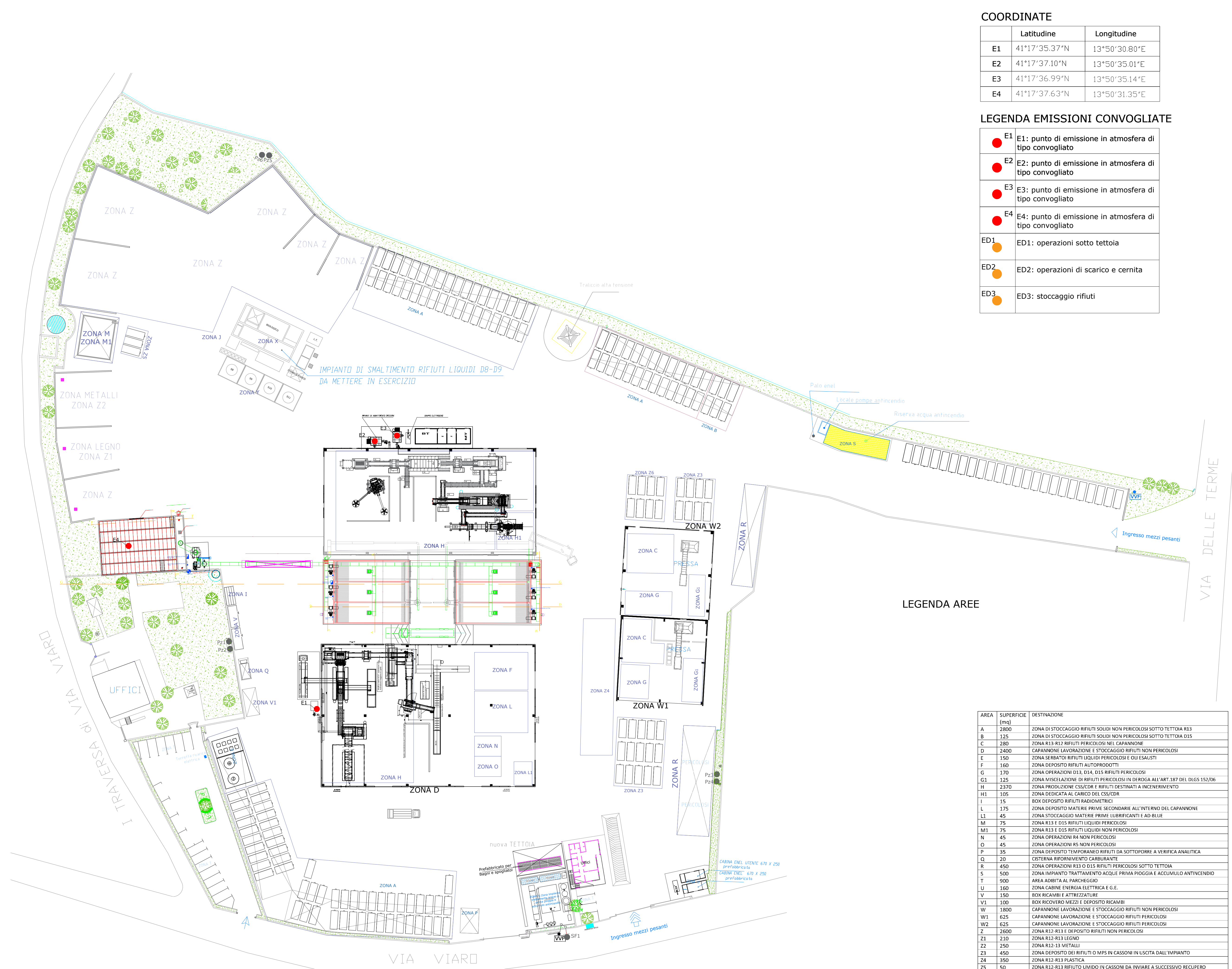
Planimetria generale rifiuti 1:500
